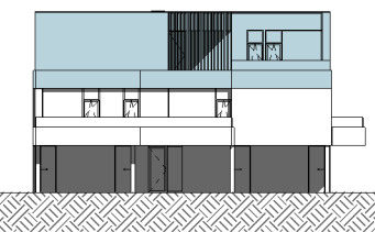
VOORGEVEL
